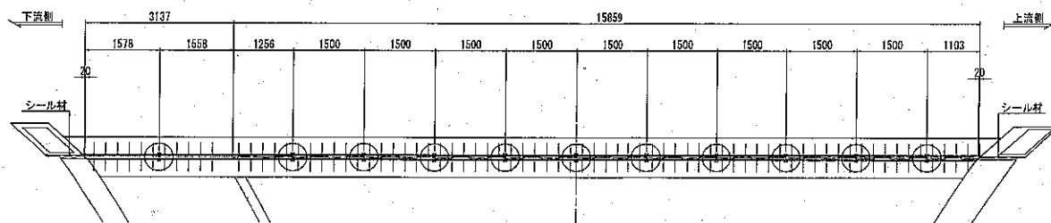
A1橋台平面図
