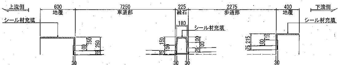
P1～P5橋脚断面図
