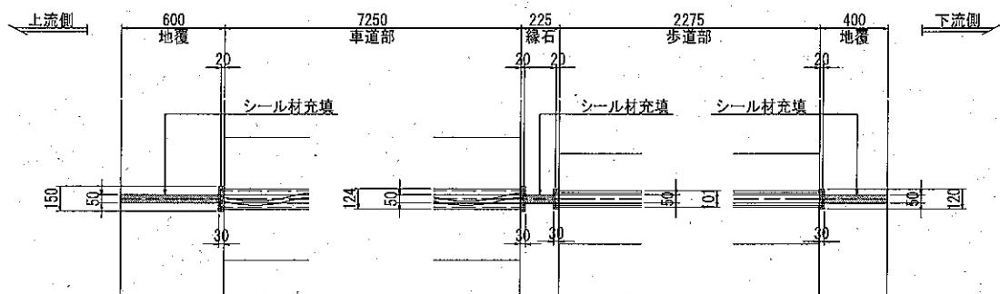
P1～P5橋脚平面図
